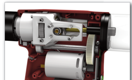
Präzisionsspindel für schnelle Setzvorgänge
